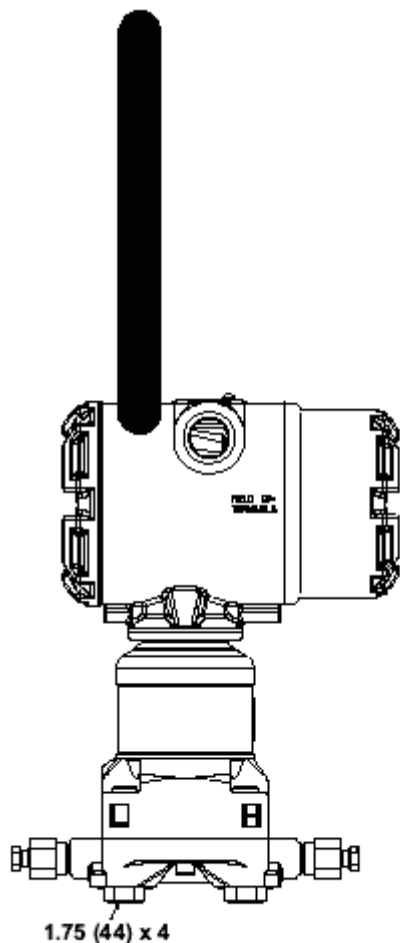
Датчик с фланцевыми болтами
