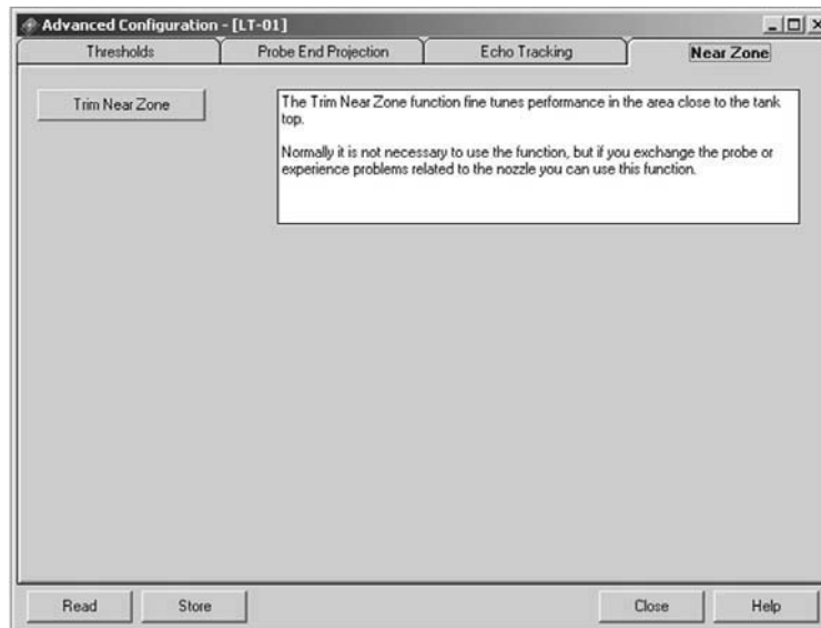
Рис. 4-1. Команда Trim Near Zone (Коррекция ближней зоны) на экране Advanced Configuration.
