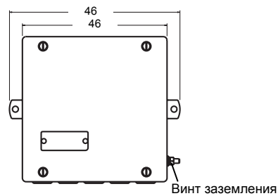
Вид спереди
