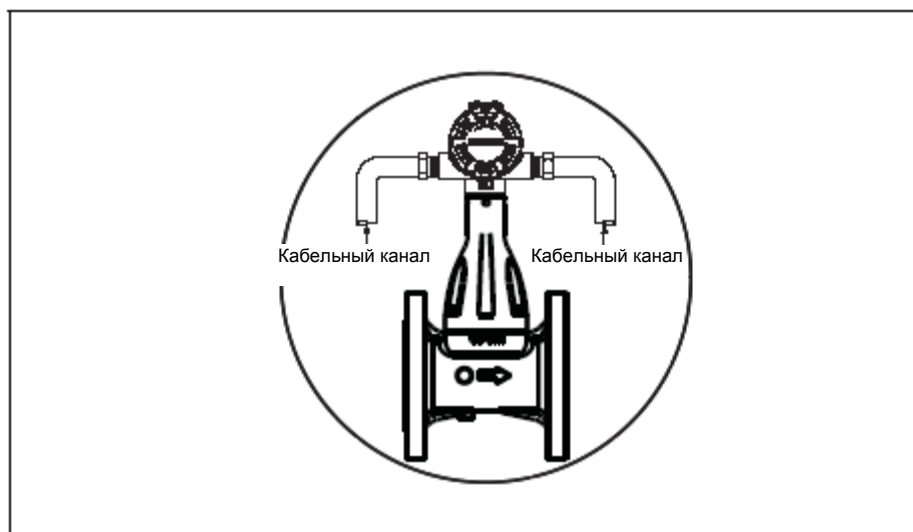
Рисунок 2-9. Правильный монтаж кабеля для расходомера
