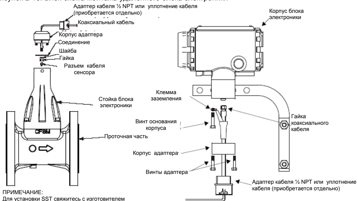
Рисунок 2-15. Блок-схема монтажа удаленного блока электроники
