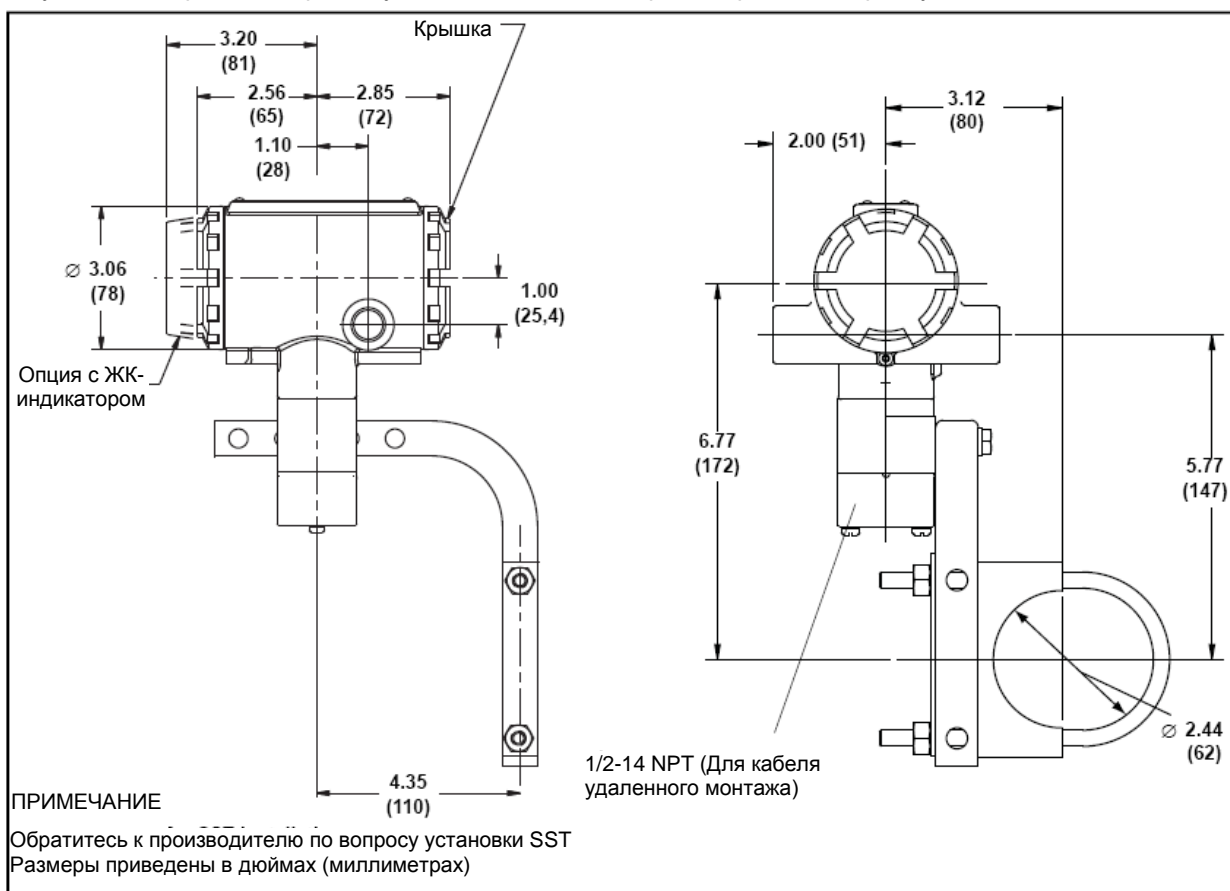
Рисунок 2. Габаритные чертежи установки блока электроники расходомера с удаленным монтажом
