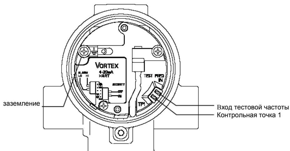
Рисунок С-2. Контрольные точки выходных сигналов вихрей (ТР1), входа тестовой частоты и клеммы заземления.
